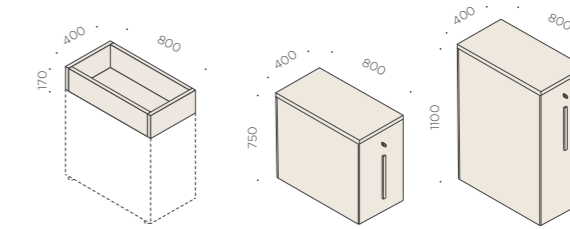
en_Planter box it_Fioriera fr_Pot à fleurs en_Low Orgatower it_Orgatower basso fr_Orgatower basse en_High Orgatower it_Orgatower alto fr_Orgatower haut
