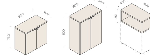
en_Side cabinet it_Contenitore laterale fr_Meuble latéral en_Side cabinet it_Contenitore laterale fr_Meuble latéral en_Open box it_Box a giorno fr_Niche ouverte
